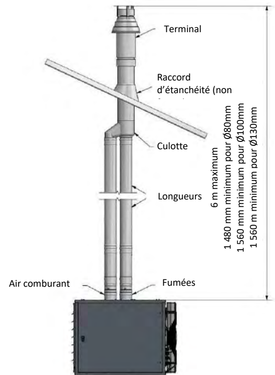
Schéma 4b Type C32 Evacuation toiture bi-tube et ventouse
