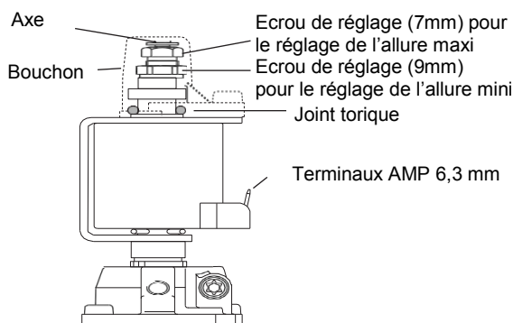
Schéma 8 Régulateur modulant
