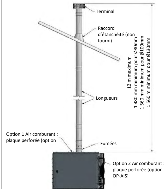
Schéma 3b Type B22 Evacuation individuelle toiture
