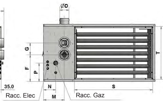
Vue arrière
