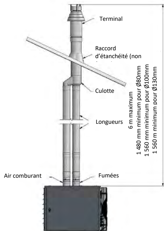
Schéma 4b Type C32 Evacuation toiture bi-tube et ventouse
