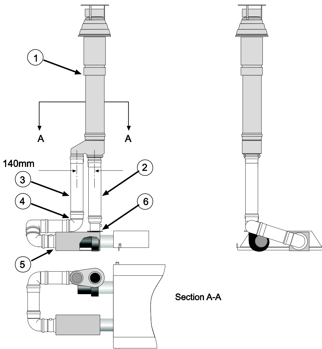
Schéma 25 Schémas de principe pour évacuation et amenée d'air avec terminal concentrique vertical
