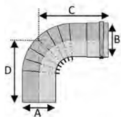
Coude 90°
